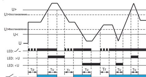
Рисунок 3.2 – Функциональная диаграмма работы
