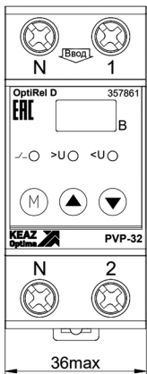
Рисунок А.1 – Габаритные размеры и маркировка реле
