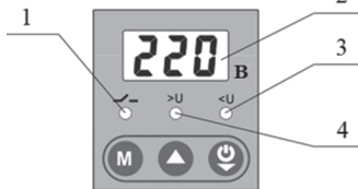
Рисунок 3.1 – Панель управления
