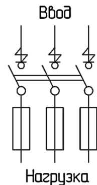
Рисунок 2. Схема электрическая принципиальная ЯРП11М-3
