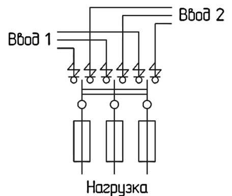
Рисунок 4. Схема электрическая принципиальная ЯРП11М-7
