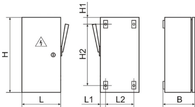
Рисунок 1. Общий вид и габаритные размеры ЯРП11М-3
