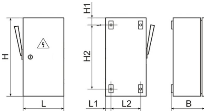
Рисунок 3. Общий вид и габаритные размеры ЯРП11М-7
