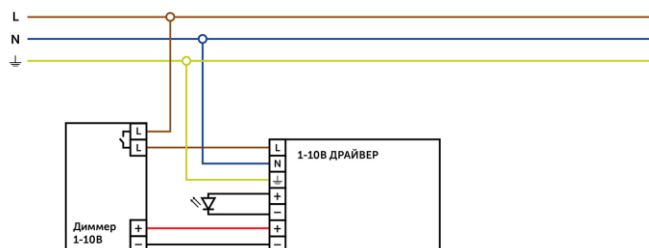
СХЕМА ПОДКЛЮЧЕНИЯ ДЛЯ ДРАЙВЕРОВ СЕРИИ LT20W 1-10V
