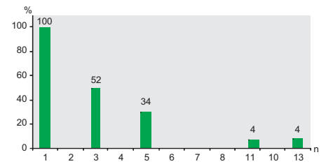
Рис. 13. Частотный спектр гармоник для однофазных промышленных устройств, индукционных печей, сварочных аппаратов, выпрямителей и пр.
