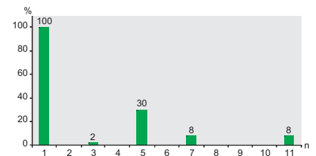
Рис. 14. Частотный спектр гармоник для трехфазных частотно-регулируемых приводов, асинхронных электродвигателей или электродвигателей постоянного тока
