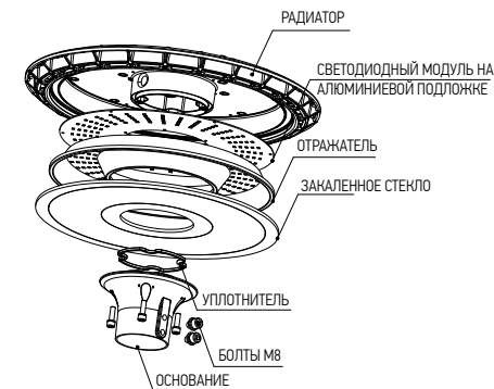
Рис.2 Взрыв-схема светильника PGL 04
