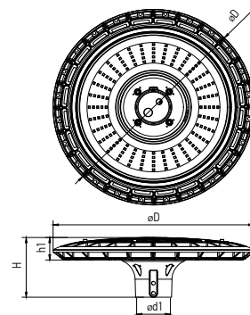
Рис.1 Светильник PGL 04
