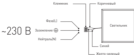
- Сүрөт.1. Кошулуу схемасы светильника тармагына 230В.
