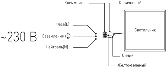
Բրինձ.1. Միացման սխեման lamp ցանցի 230V.
