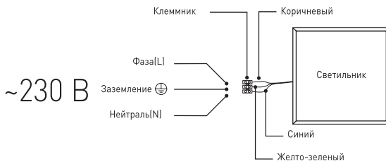
Сурет: 1. Шамды 230В желіге қосу схемасы.
