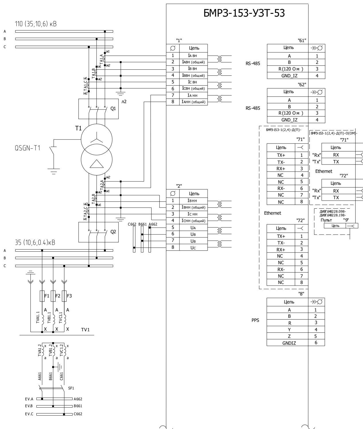
Рисунок А.1 - Схема электрическая подключения при использовании трех ТТ со стороны НН
