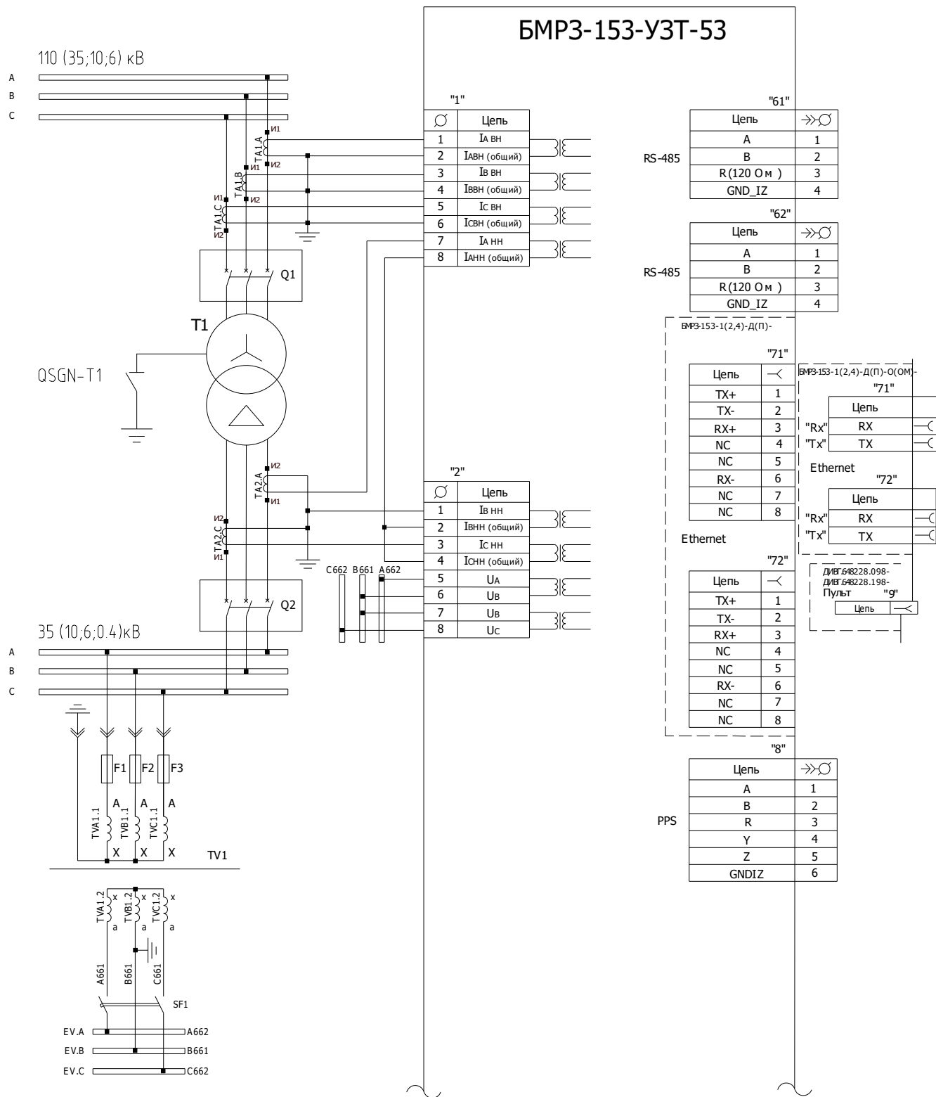
Рисунок А.2 - Схема электрическая подключения при использовании двух ТТ со стороны НН
