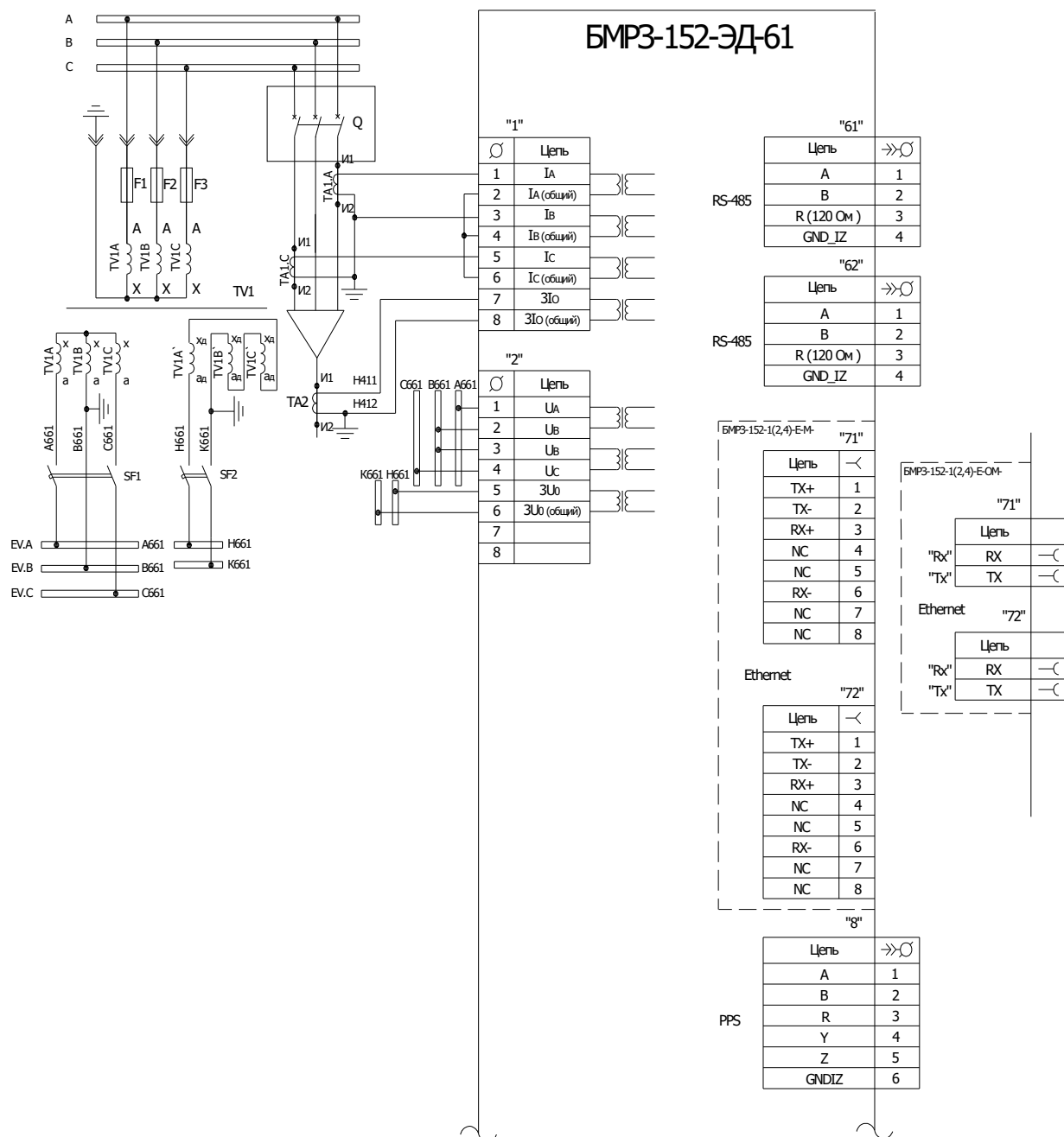
Рисунок А.2 - Схема электрическая подключения (два трансформатора тока)
