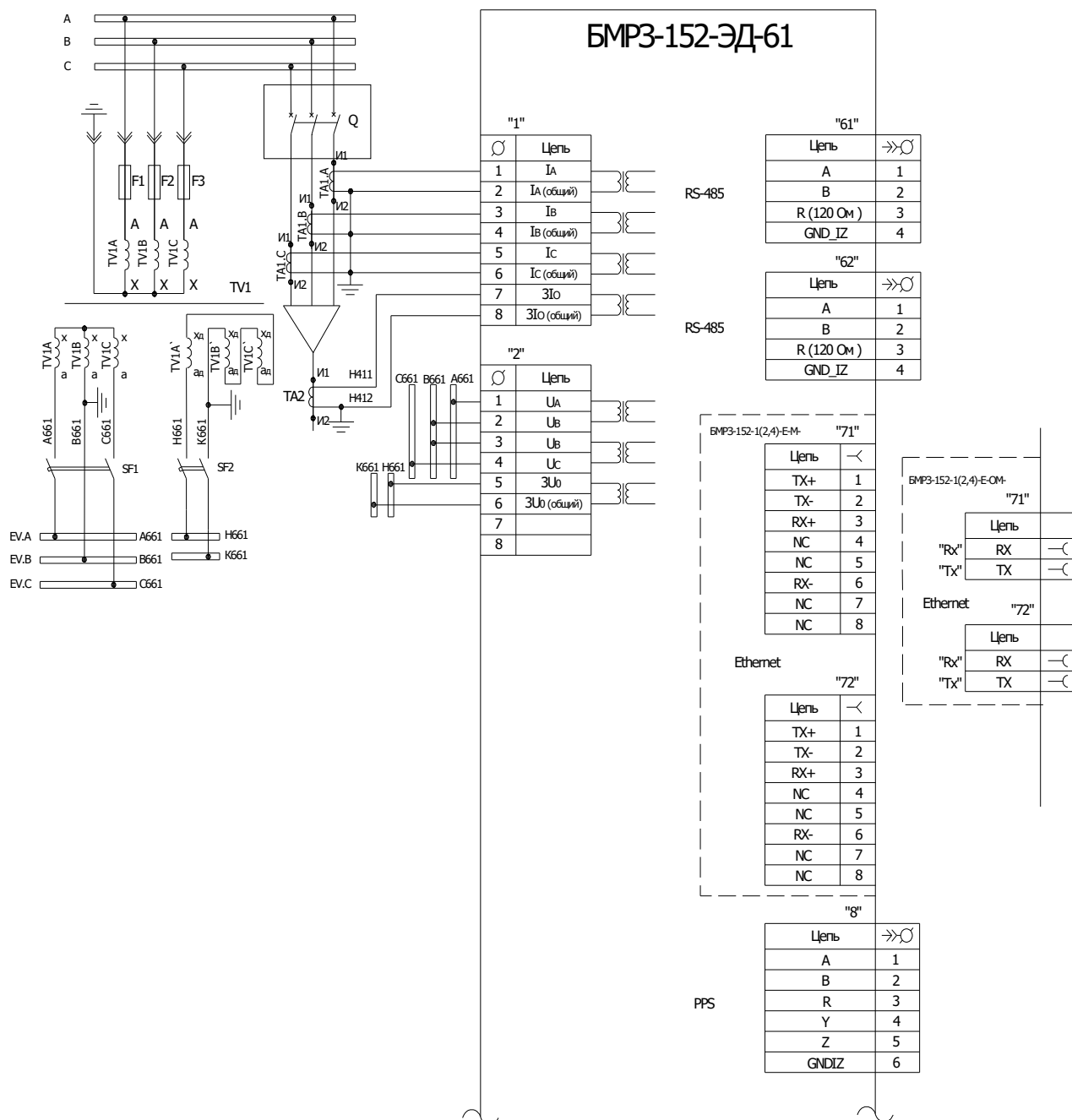
Рисунок А.1 - Схема электрическая подключения (три трансформатора тока)
