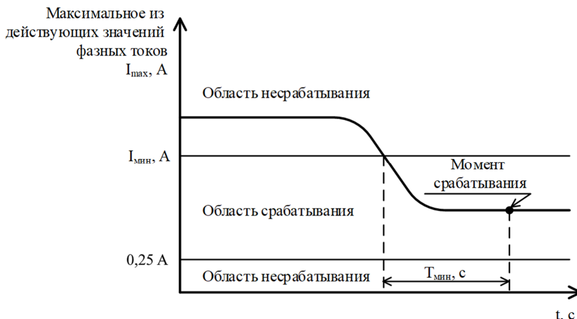
Рисунок 3 - Условия срабатывания Мин. ТЗ
