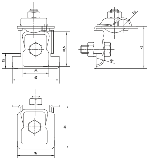
Рисунок 1 – Габаритные размеры
