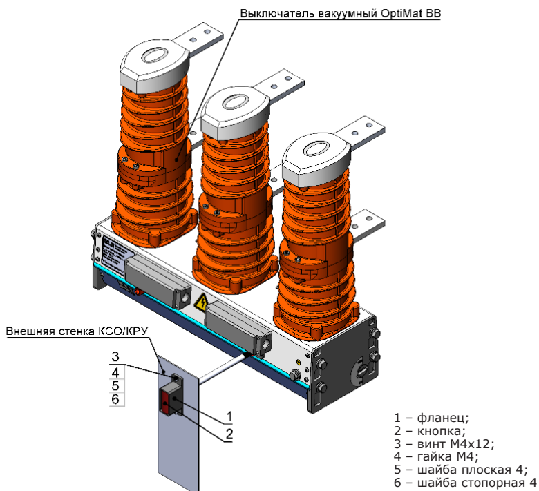
Рисунок А.1 – Пример условного монтажа комплекта КМ-04
