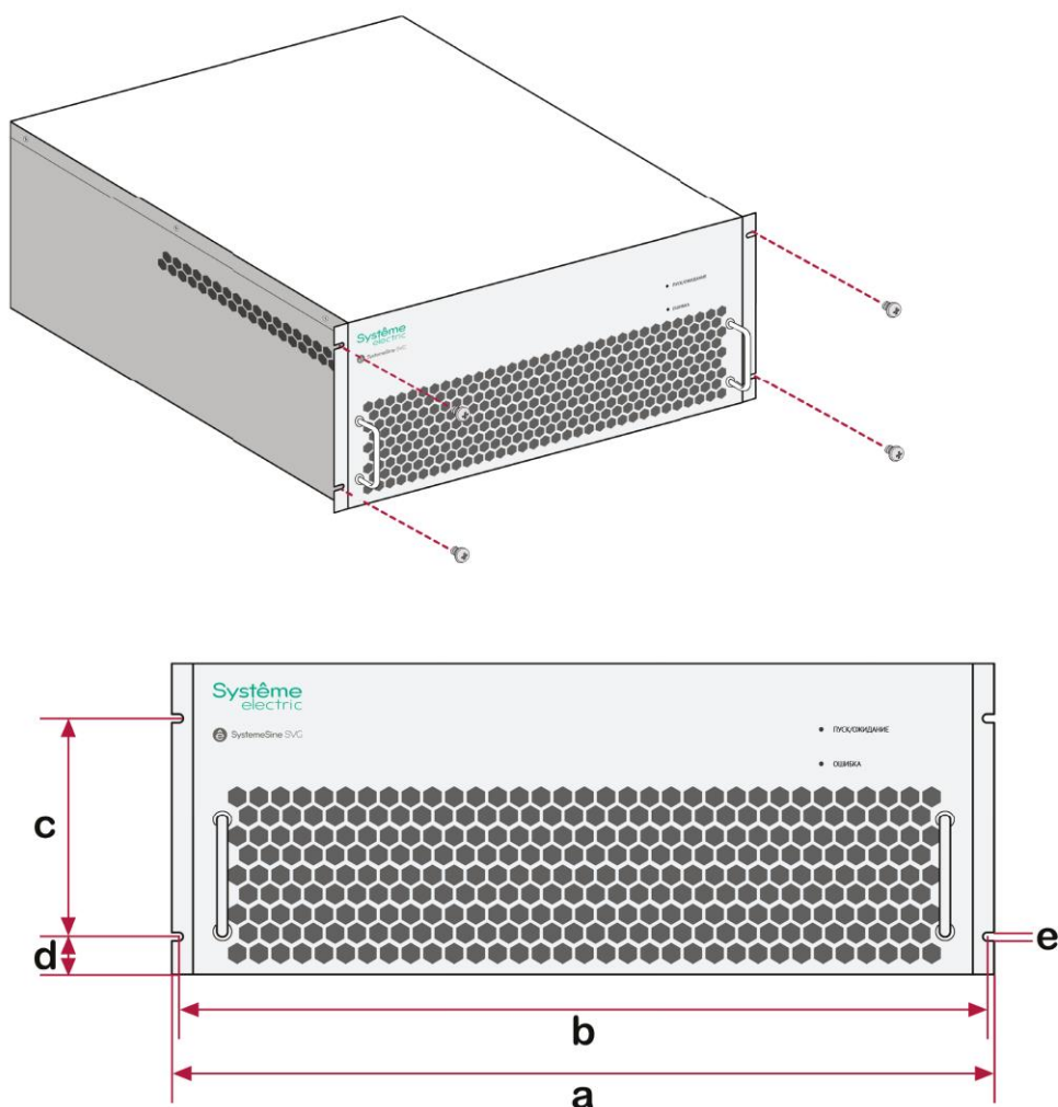
Рис. 5.5.1.1 Монтаж стоечного модуля IP20 (вид спереди)
