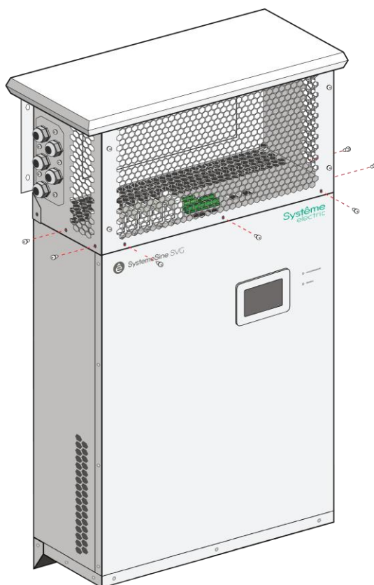
Рис. 5.5.3.1 Крепление влагозащитного комплекта IP31 к модулю СГРМ
