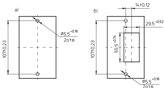
Рисунок Б.4 - Сверление отверстий под винты крепления двухполюсного выключателя: а) на панель; б) за панелью
