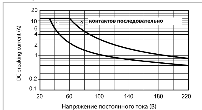
H 56 - Макс. отключающая способность DC1 Версия с контактами NO
