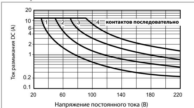
H 56 - Макс. отключающая способность DC1 Версия с контактами CO
