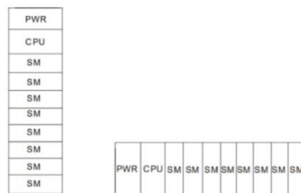
Варианты установки модуля контроллера (CPU) совместно с модулем питания (PWR) и модулями расширения (SM): а) вертикально, б) горизонтально
