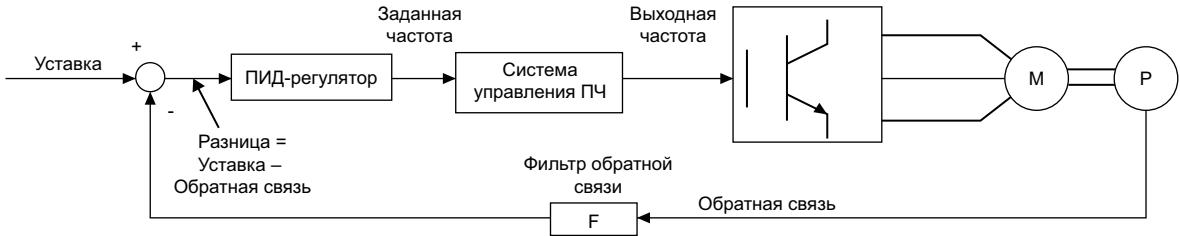
Рисунок 4-24 Блок-схема ПИД-регулирования
