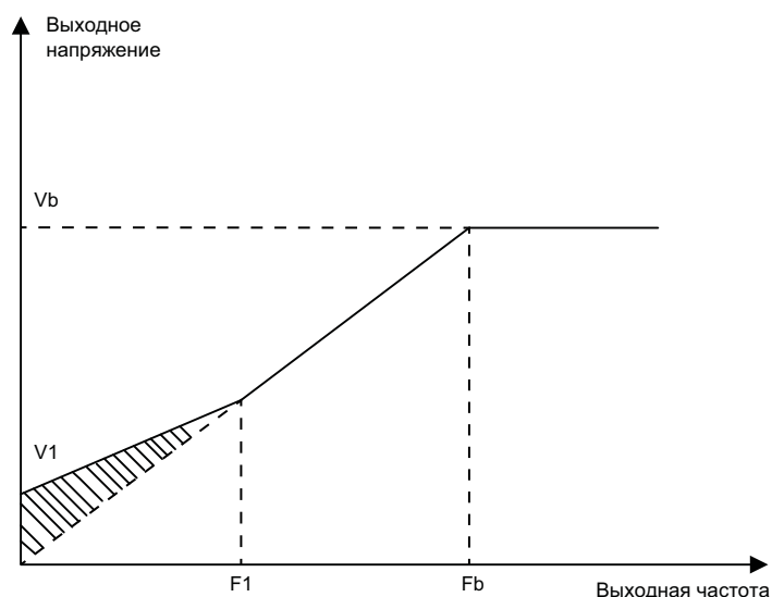
Рисунок 4-2 Форсировка момента
