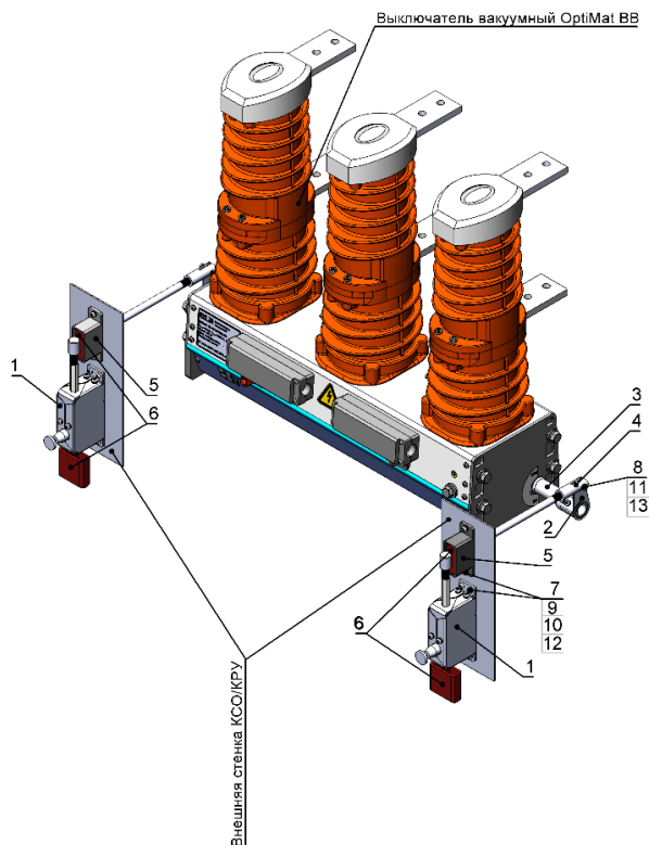
Рисунок А.1 – Пример условного монтажа комплекта КМ-06
