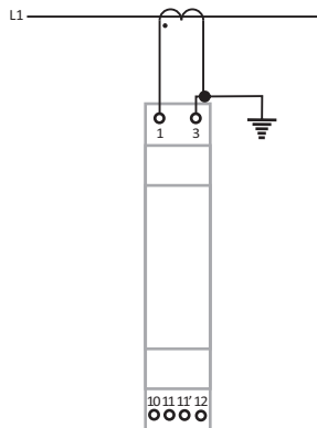
Косвенное измерения тока с использованием трансформаторов тока.
