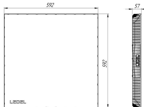
Рисунок 1 Светильник «L-office 32 Premium»
