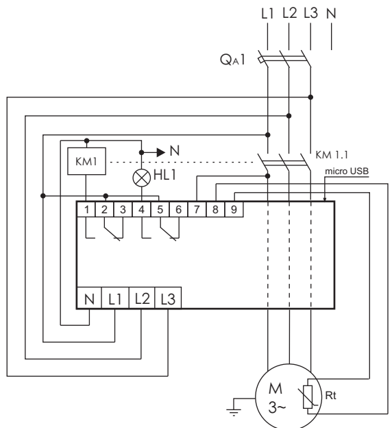
Рисунок 2 - Типовая схема включения AZD-M.
