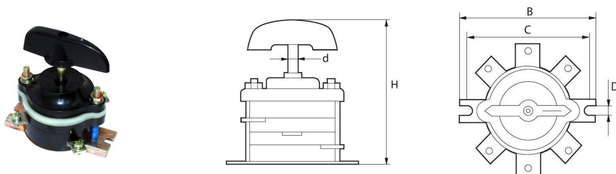
Пакетные выключатели со степенью защиты IP00, крепление – задней скобой
