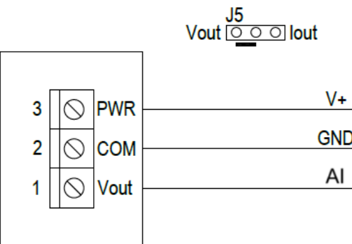
Подключение по трехпроводной схеме (сигнал 0...10 В) к аналоговому входу контроллера
