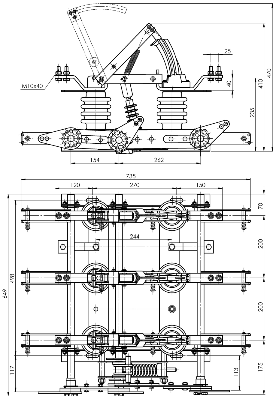
Рисунок А.5 – Выключатель нагрузки автогазовый типа ВНА-10/630-Л-IIIз-И2-УХЛ2
