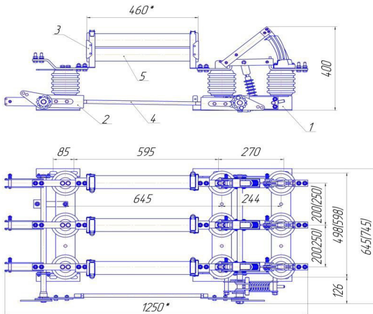
Рисунок А.1 - Выключатель нагрузки автогазовый типа ВНА-10/630-П-з-И2-УХЛ2, масса не более 35 кг
