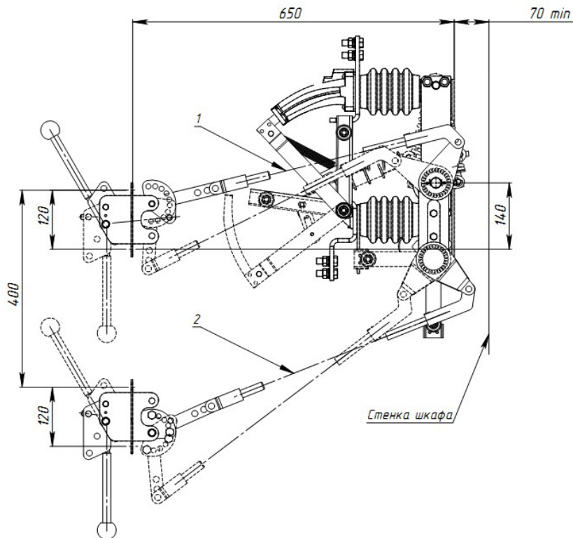
Рисунок 3 – Возможный монтаж трехполюсного выключателя с приводом ПРБД-10
