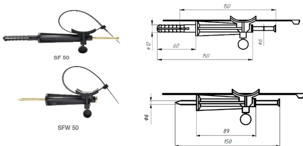
Рис. 1. Внешний вид фасадных креплений SF 50, SFW 50.
