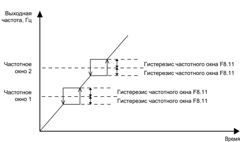
Рисунок 4-17 Логика работы функции частотного окна во время разгона и торможения
