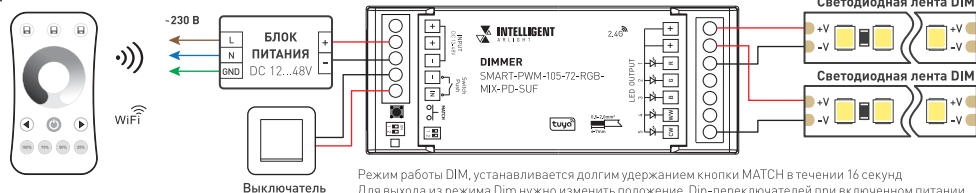
Рис. 1. Схемы подключения диммера SMART-PWM-105-72-RGB-MIX-PD-SUF
