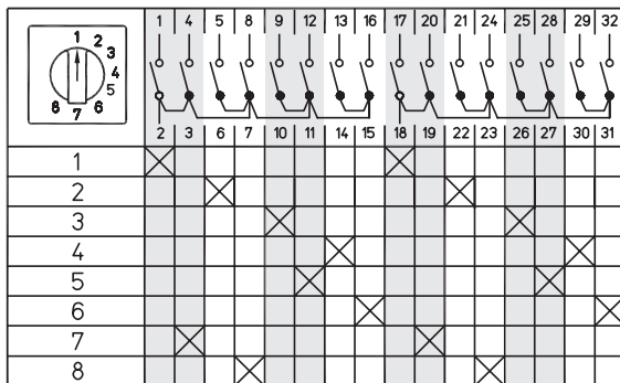
2-полюсные, 8 позиций Схема 118
