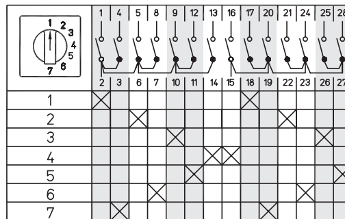
2-полюсные, 7 позиций Схема 117
