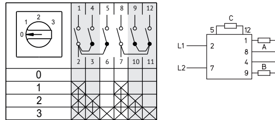
2-полюсные 3-групповые Схема 255
