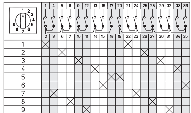
2-полюсные, 9 позиций Схема 119
