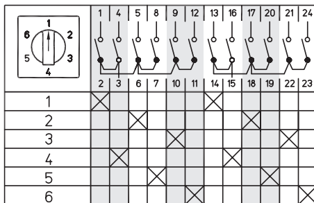
2-полюсные, 6 позиций Схема 89
