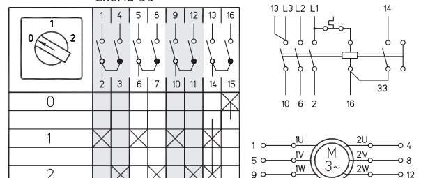
С управлением контактором Схема 33
