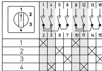
2-полюсные, 4 позиции Схема 87
