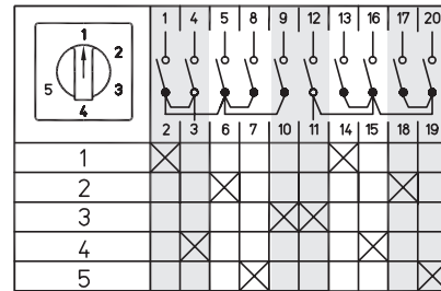
2-полюсные, 5 позиций Схема 88
