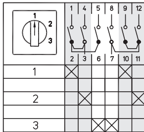
2-полюсные, 3 позиции Схема 86
