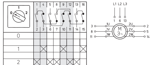
Двухскоростные 0- \Delta - \Upsilon\Upsilon Схема 19
