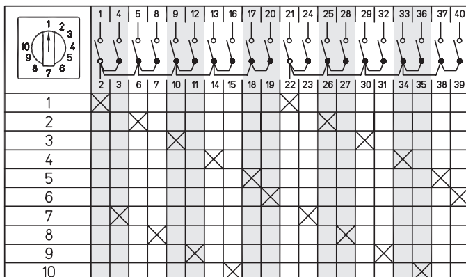
2-полюсные, 10 позиций Схема 120
