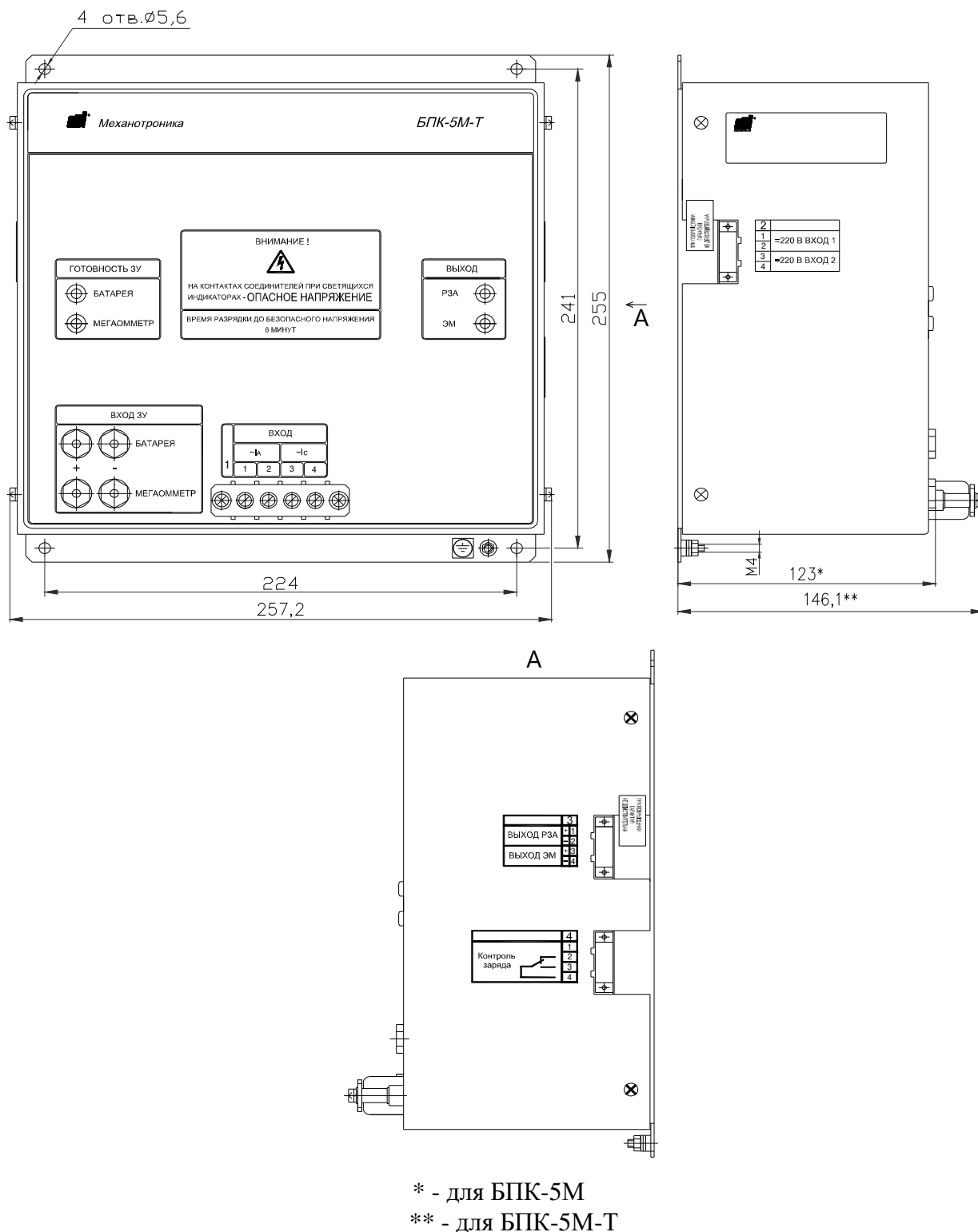
Рисунок 1 - Габаритные и установочные размеры БПК
