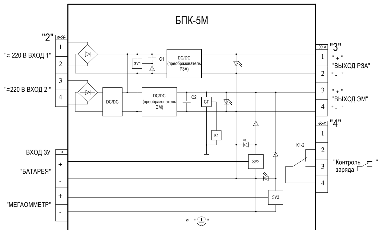
б) схема БПК-5М
