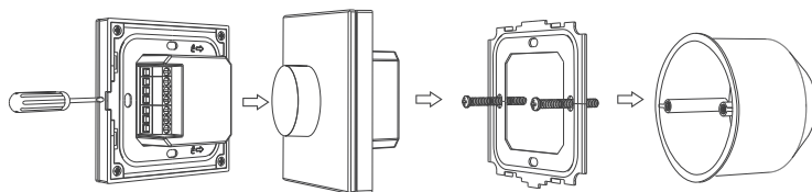
Рисунок 3. Монтаж панели
