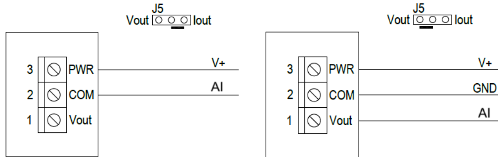
Подключение по двухпроводной схеме сигнала 4...20 мА к аналоговому входу контроллера
