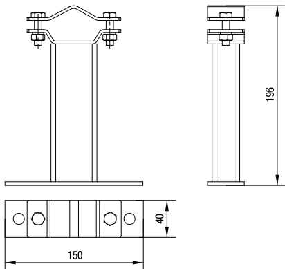
Рисунок 1 – Габаритные размеры
