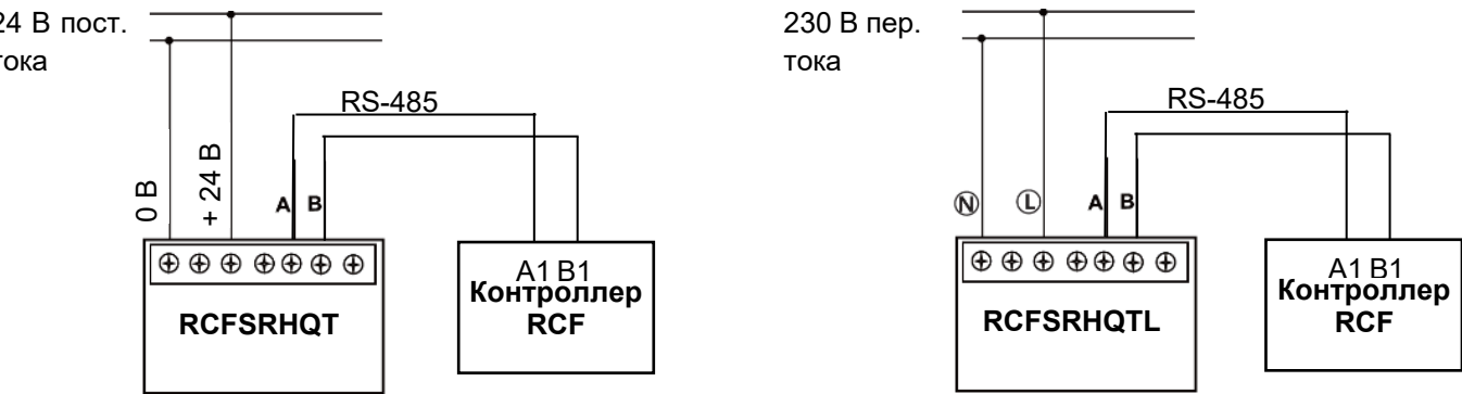
Схема подключения датчиков RCFSRHQT, RCFSRHQTL
