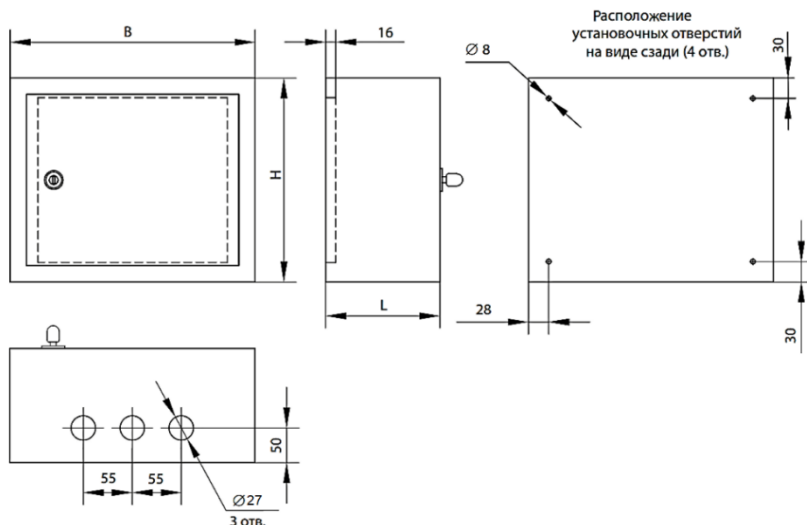
Рисунок 1. Габаритные и установочные размеры ящика управления освещением
