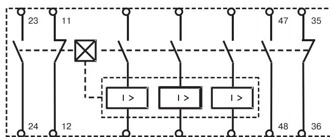
Трехполюсный автоматический выключатель с 2 размыкающими и 2 замыкающими контактами
