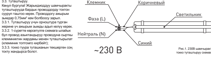
Рис.1. Схема подключения светильника к сети 230В.
