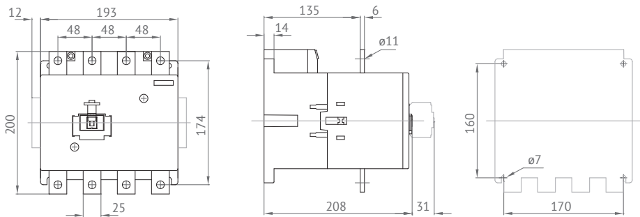
Контакторы четырехполюсные AC
