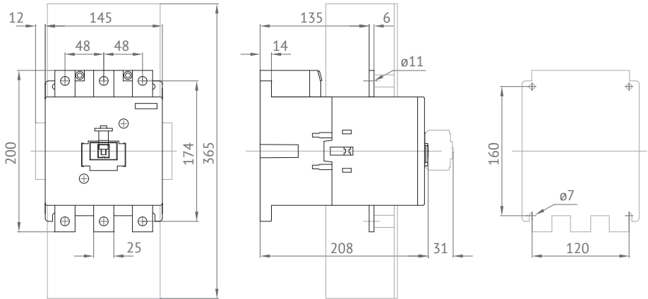
Контакторы трехполюсные AC/DC
