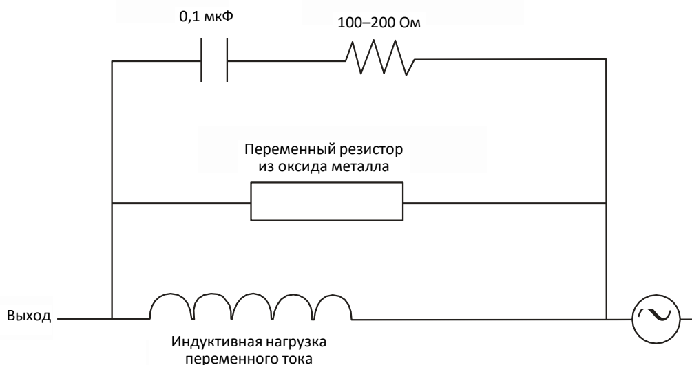
Рисунок 1-6. Цепь подавления нагрузки переменного тока
