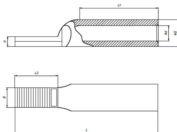
Рис. 1. Внешний вид наконечников типа НШЛ.
