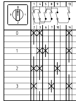
1-полюсные 0-1-2-3 Схема 98
