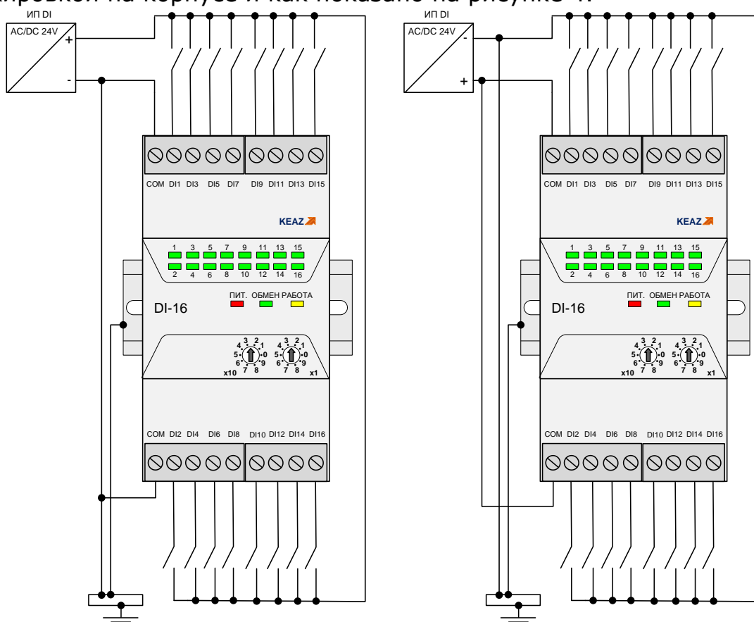
Рисунок 4 – Схемы подключения модуля
