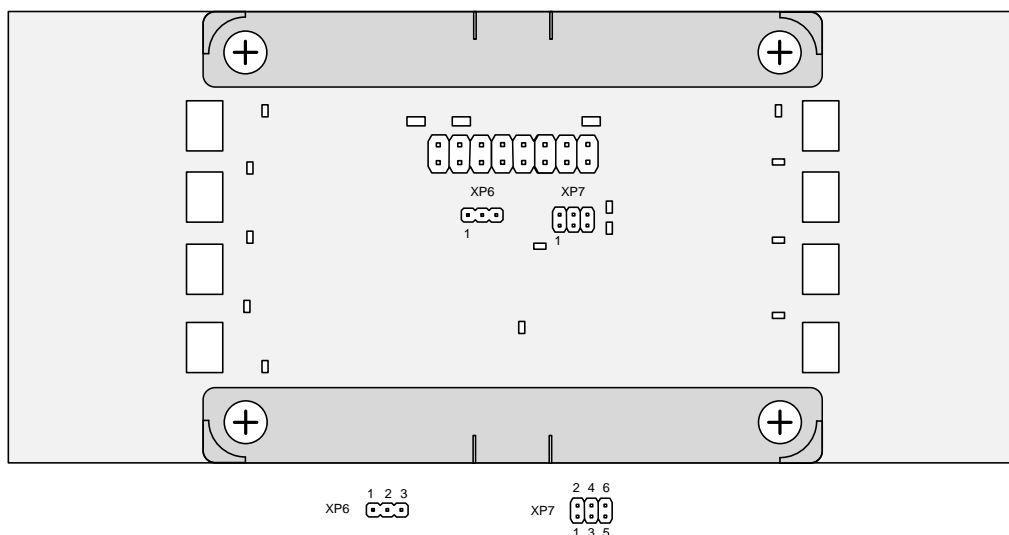
Рисунок 3 – Расположение перемычек XP6 и XP7
