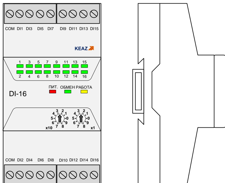
Рисунок 1 – Внешний вид и размеры модуля
