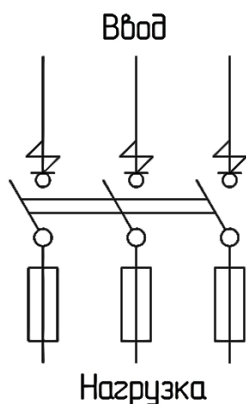
Рисунок 1. Принципиальная электрическая схема силовых ящиков серии ЯВЗ.
