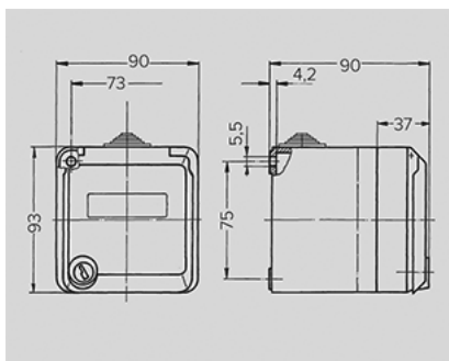
Чертеж 1 МВ 564 Размеры, мм.
