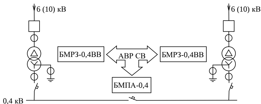
Рисунок 4 - Структурная схема АВР
