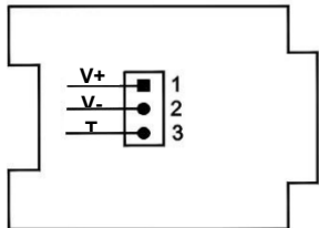
0...10 В пост. тока 3-проводная схема
