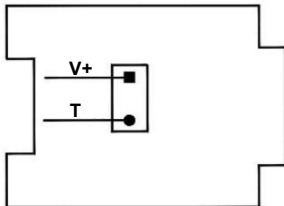
4...20 мА 2-проводная схема
