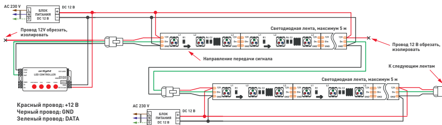
Рис. 3. Схема подключения нескольких светодиодных лент SPI-B60 и SPI-SE-B60 с двух сторон с использованием SPI-контроллера с одним выходным портом и отдельных блоков питания
