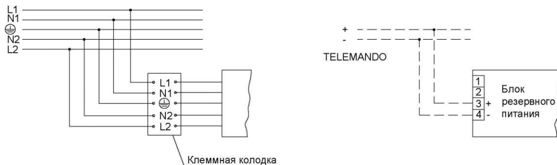
Схема электрических соединений
