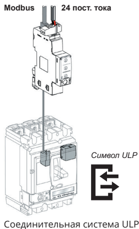
Соединительная система ULP
