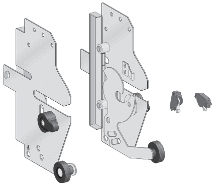
Неподвижная часть шасси
