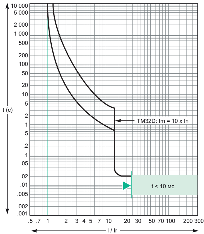
TM32D
