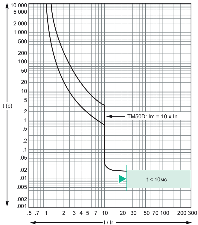
TM50D
