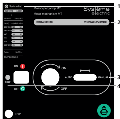
Выключатель с мотор-редуктором
