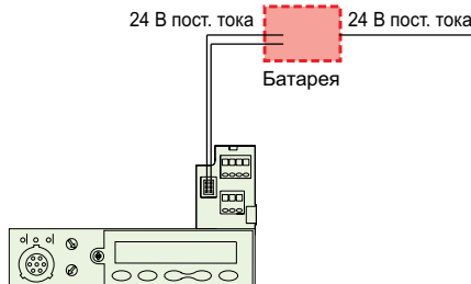
Модуль питания без функции передачи данных, через клеммник с резервной батареей
