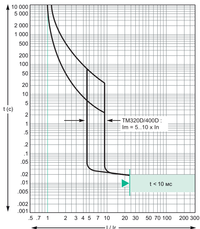
TM320D/TM400D
