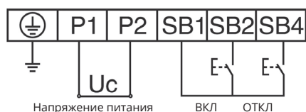
Схема подключения мотор-редуктора
