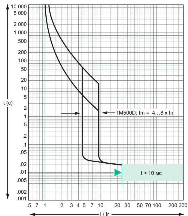
TM500D
