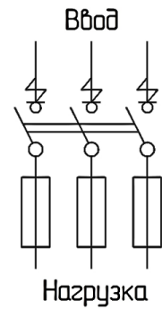
Рисунок 2. Схема электрическая принципиальная ЯВЗ
