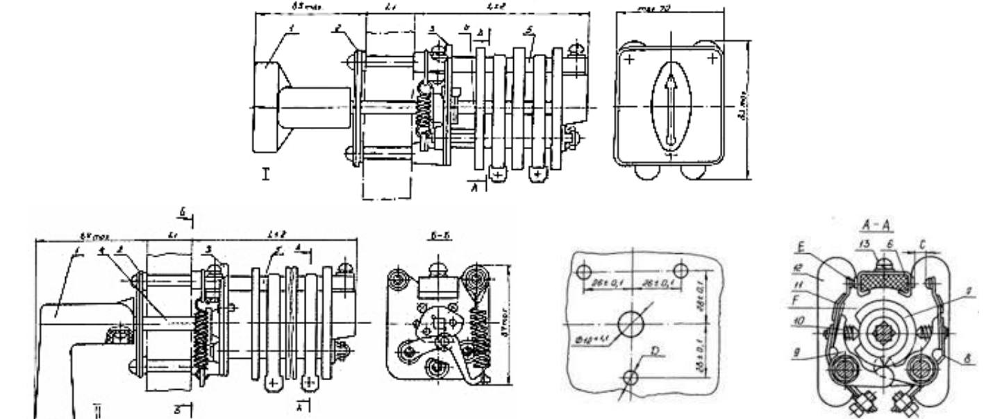
Рисунок 1. Габаритные и установочные размеры пакетных переключателей I - с фиксацией рукоятки; II - с самовозвратом рукоятки; L - длина набора секций; L1 -толщина панели; D - 3 отв. диаметром 6 мм; E - нажатие контактов (не менее 0,1 кг); F - провал (не менее 0,7 мм); C - раствор контактов (не менее 6 мм)
