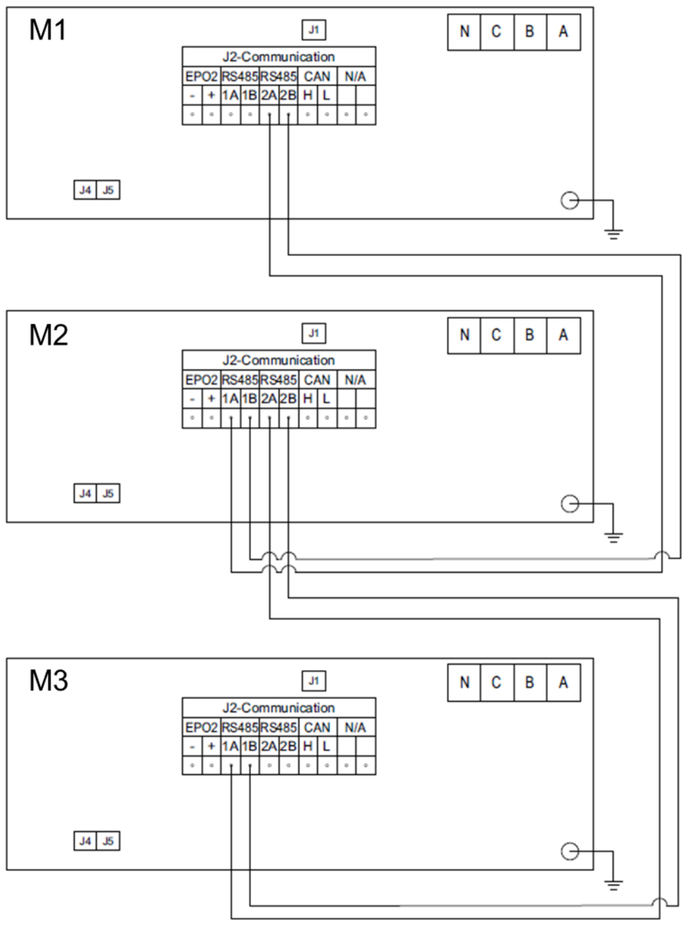
Рис. 6.4.2.3 Подключение RS485 при параллельном режиме работы
