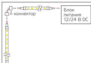
Рис. 1. Подключение коннектора
